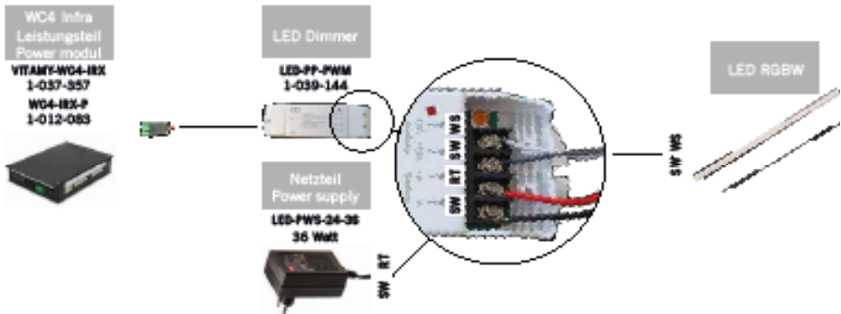
Abb. 27: Verbinden des LED RGBW mit der Steuerung
