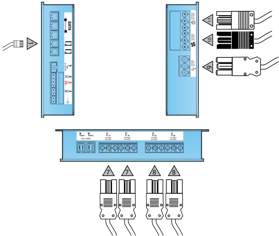
Abb. 26: Anschlüsse Leistungsteil
