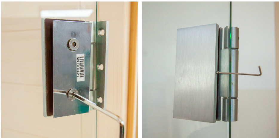
Abb. 32: Montage Türbeschläge 2
