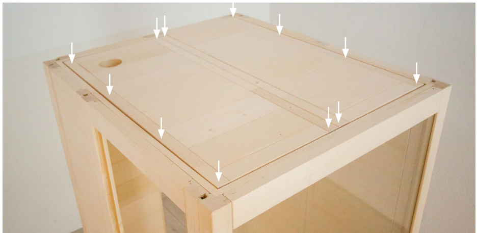
Abb. 15: Befestigen der Dachelemente
